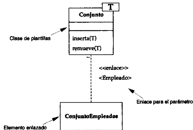
Figura 5-17: Elemento enlazado (versión 2)
