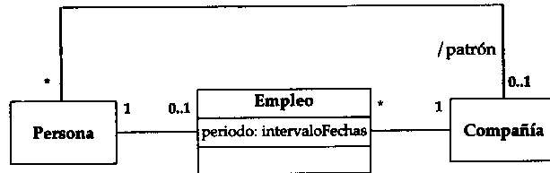
Figura 5-12: Promoción de una clase de asociación a una clase completa
