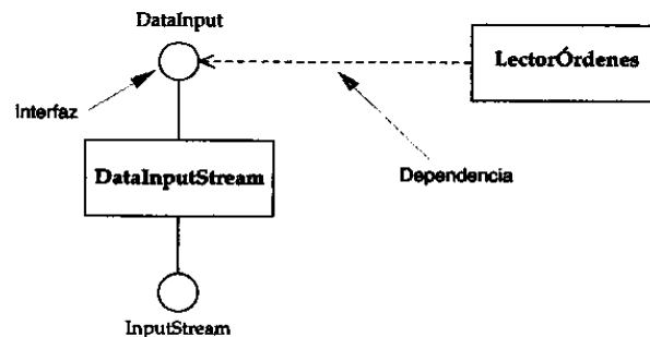
Figura 5-9: Notación de paletas para representar interfaces
