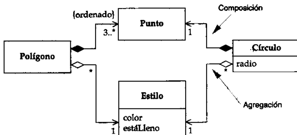
Figura 5-3: Agregación y composición
