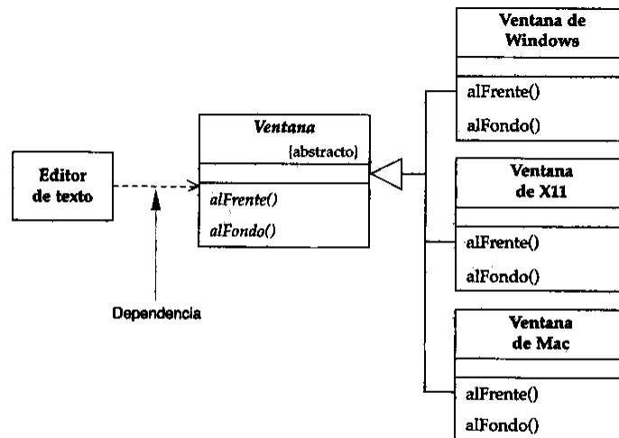
Figura 5-7: Ventana como clase abstracta
