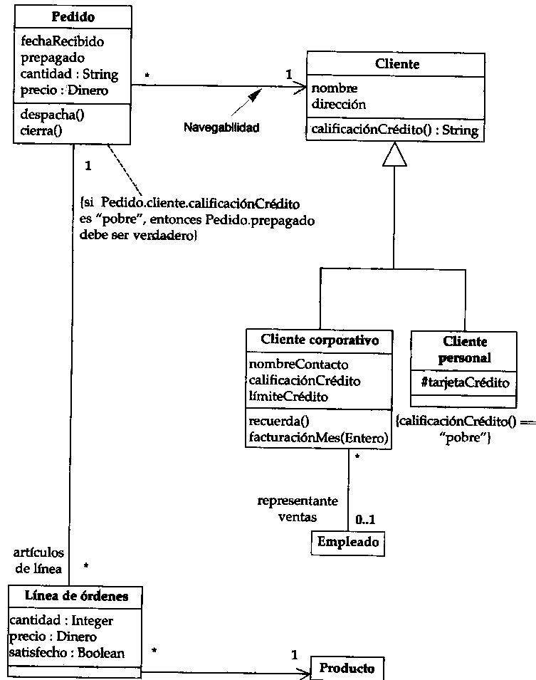
Figura 4-3: Diagrama de clase con navegabilidades
