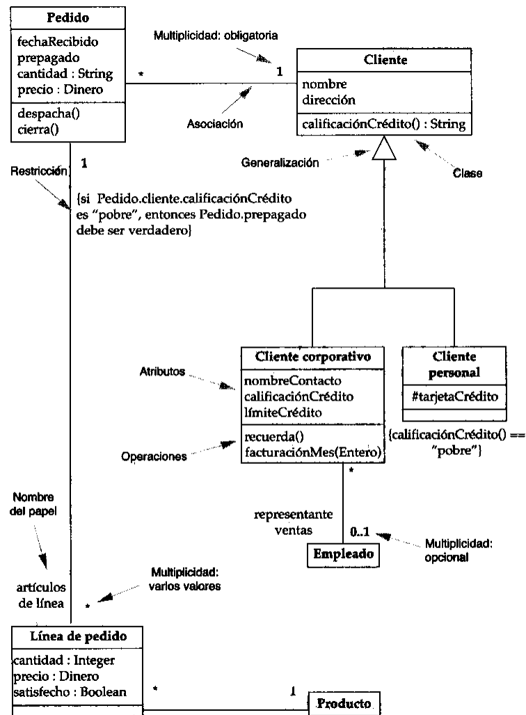
Figura 4-1: Diagrama de clase
