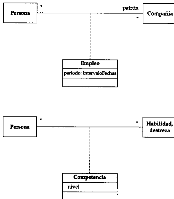
Figura 5-13: Sutilezas de la clase de asociación
