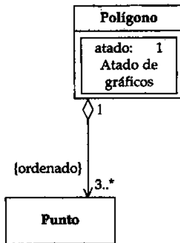
Figura 5-4: Notación alterna para la composición
