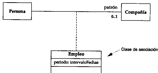
Figura 5-11: Clase de asociación
